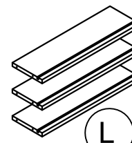
3 drawer backs 3 traseros del cajon 3 dos de tiroir 37243302120
