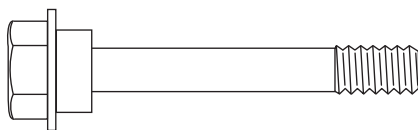
(6) VIS À ÉPAULEMENT 1/4-20 x 1-3/4
