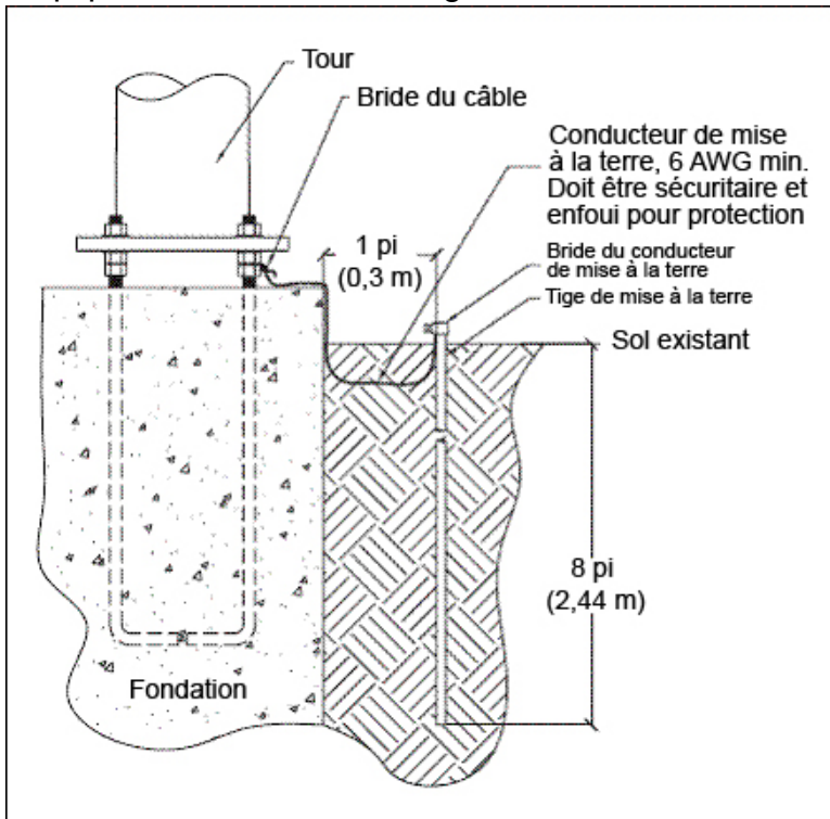
Exemple de mise à la terre d'une éoliennet
