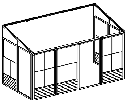
D-3 FRAME
