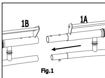
Fig. 1, Fig. 2 : Insérez chaque bâti de gauche (1A) dans le bâti de droite (1B) pour former quatre écrans latéraux et fixez-les à l'aide des vis AA et des rondelles BB.
