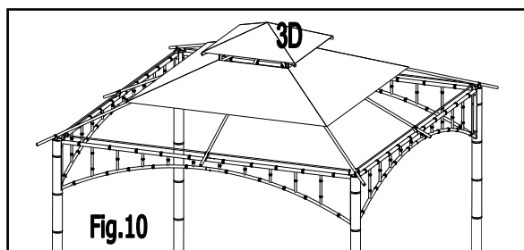
Fig. 10 : Installez la toile du toit (3D).
