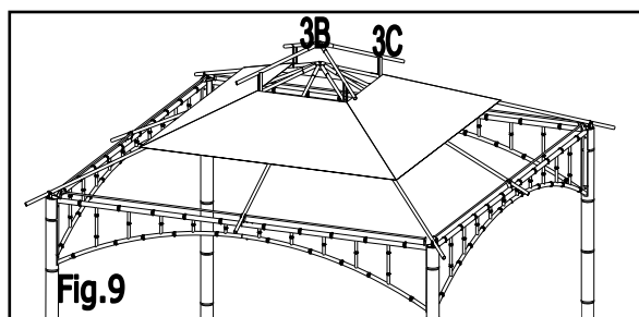
Fig. 9 : Insérez la petite barre supérieure (3C) dans le raccord du toit (3B). Utilisez ensuite les vis CC, les rondelles BB et les écrous DD pour fixer la petite barre supérieure (3C) et les barres du deuxième toit.
