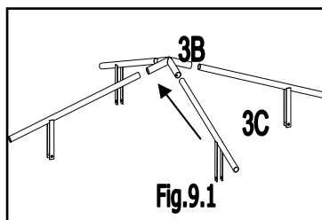
Fig. 9 : Insérez la petite barre supérieure (3C) dans le raccord du toit (3B). Utilisez ensuite les vis CC, les rondelles BB et les écrous DD pour fixer la petite barre supérieure (3C) et les barres du deuxième toit.
