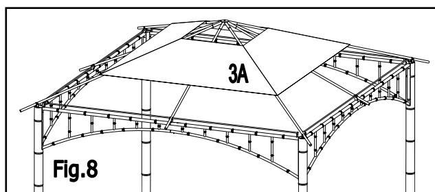
Fig. 8 : Placez la toile du deuxième toit (3A) sur le dessus du toit. Vous devez assembler le deuxième toit avant d'avoir terminé.
