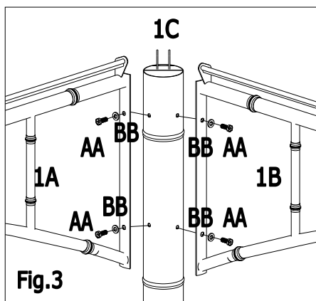
Fig. 3 : Complétez la structure en fixant les écrans assemblés sur quatre colonnes (1C) à l'aide des vis AA et des rondelles BB.
