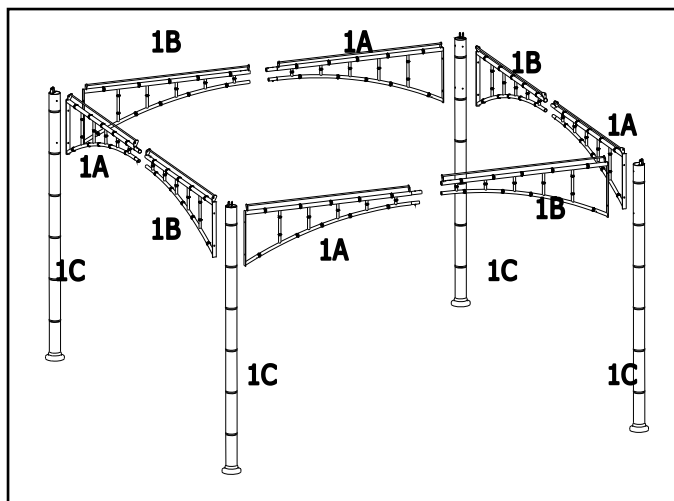
Fig. 3 : Complétez la structure en fixant les écrans assemblés sur quatre colonnes (1C) à l'aide des vis AA et des rondelles BB.
