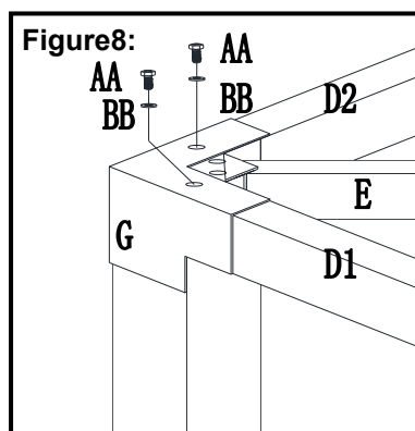
Figure8: Fixez le Fleuron du coin (G) avec boulon (AA), joint (BB) dans sa position du coin.
