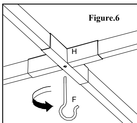
Figure.6: Fixez le crochet (F) à la connexion du toit (H).
