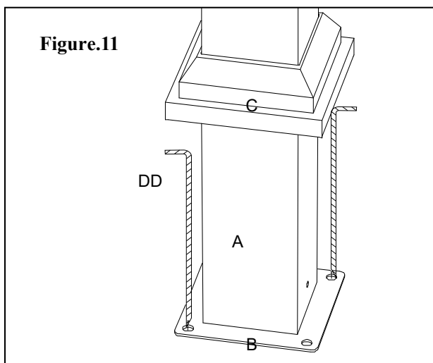
Figure.11: Fixez la pergola assemblée à la terre avec les piquets (DD).
