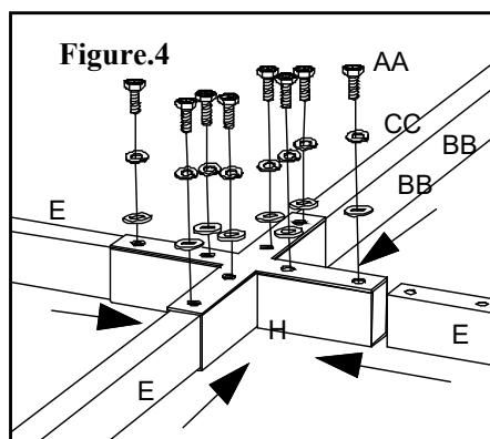
Figure.4: Fixez la Poutre inclinée (E) à la connexion du toit (H), fixez-les avec boulons (AA), rondelles à ressort (CC) et rondelles (BB), ne les serrez pas tout à fait.
