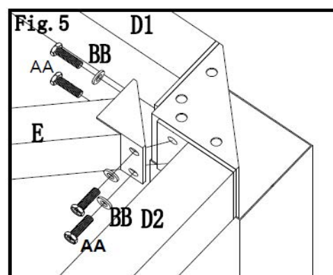
Figure.5: Fixez les poutres inclinées (E) assemblées à la colonne avec boulons (AA), rondelles (BB) et traverse (D1/D2).
