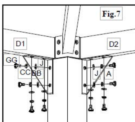
Figure.7: Support d'angle attaché (J) au poteau (A) et à la traverse 1/2 (D1 / 2) par boulon (GG), rondelle élastique (CC) et rondelle (BB). Plaidoyer.
