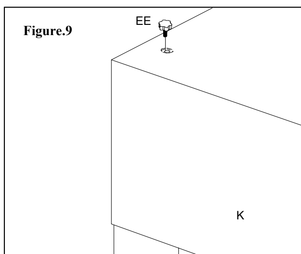
Figure.9: Placez la Toile (K) sur le toit de la Pergola, ensuite fixez chaque coin avec le Bouton d'aplomb (EE).
