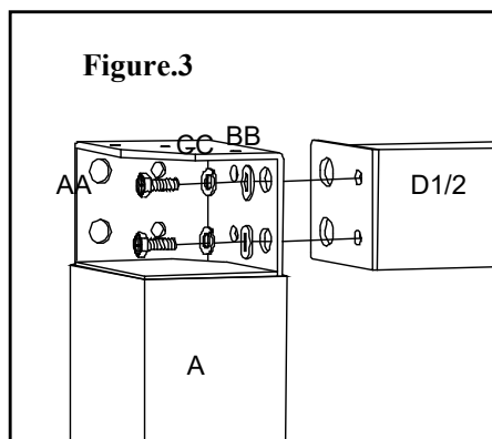
Figure.3: Fixez les Traverses 1/2 (D1/2) au Poteau (A) avec Boulon (AA), rondelles à ressort (CC) et rondelles (BB). Plea.
