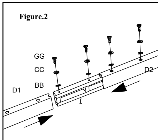
Figure.2: Fixez la Traverse1 (D1) et la Traverse 2 (D2) à la connexion des poutres (I) avec boulons (GG), Rondelles à ressort (CC) et les rondelles (BB). Plea.
