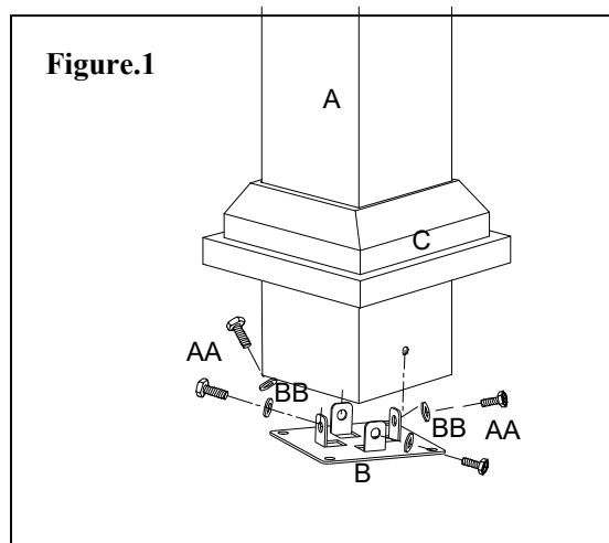
Figure.1: Introduisez le couvert de la base (C) dans le Poteau (A), et fixez la base (B) à la partie inférieure du poteau (A) avec les boulons (AA) et les rondelles (BB)
