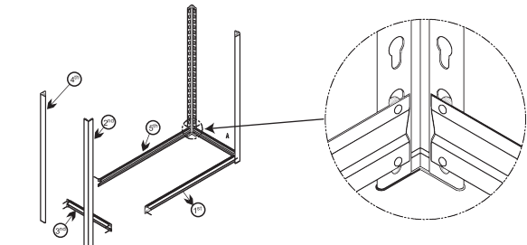
Étape 2 - Assemblage du cadre inférieur
