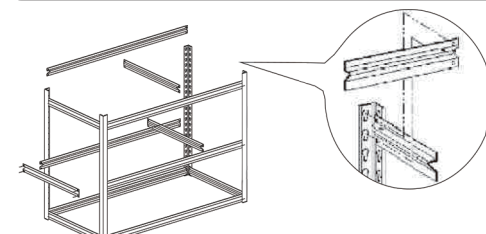
Étape 3 - Ajout de la traverse Z supérieure
