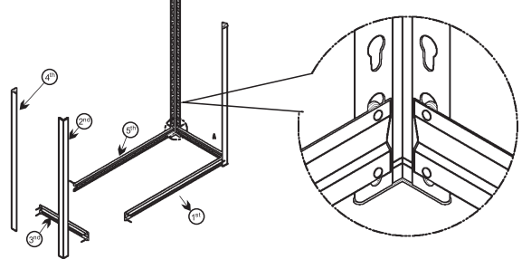
Étape 2 - Assemblage de l'unité principale
