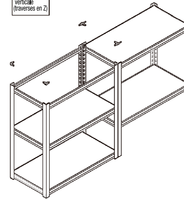
Étape 7 - Joindre les cadres (étape facultative)
