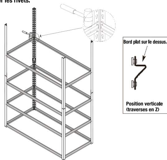
Étape 6 - Renforcement de la section supérieure
