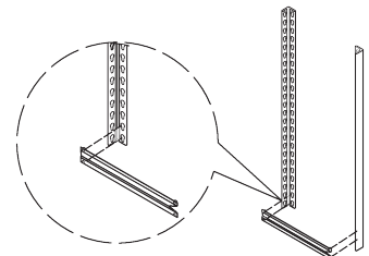
Étape 1 - Assemblage de l'extrémité inférieure
