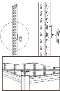
Étape 7 - Joindre les cadres (étape facultative)
