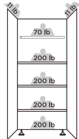
Armoire haute de 30 po 892 lb (405 kg) max.
