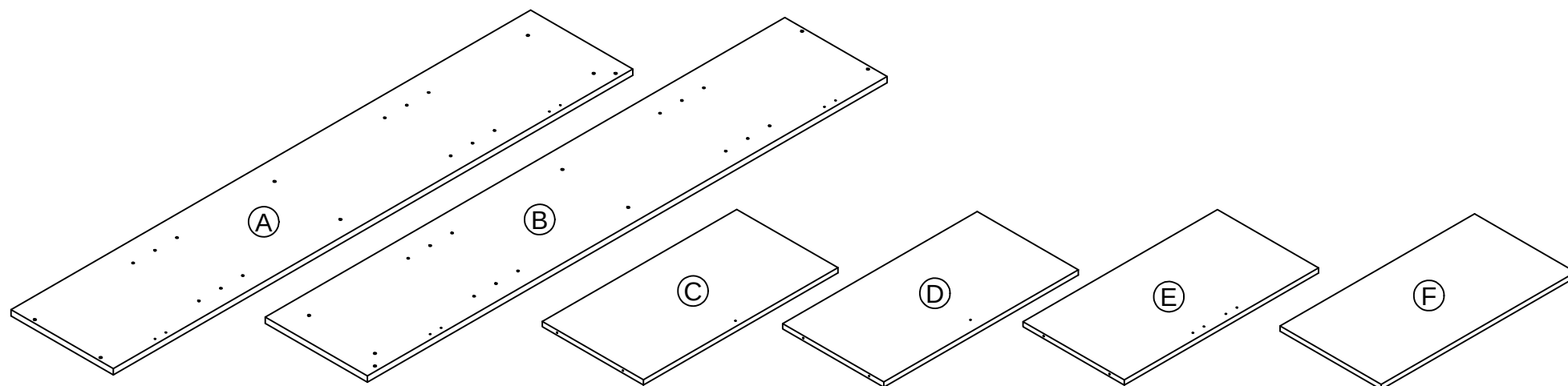
left panel panel izquierdo panneau gauche 37391015010
