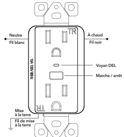
Diagramme du câblage
