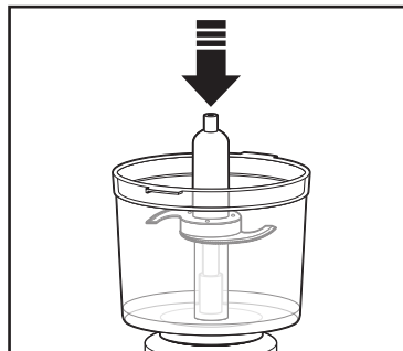
3. Glisser soigneusement la lame sur l'arbre du moteur.
