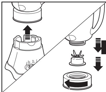
2. Quite la jarra de la licuadora de la base. Gire el collar en sentido de las agujas del reloj hasta que el collar y el conjunto de cuchillas de corte se separen de la jarra de la licuadora.
