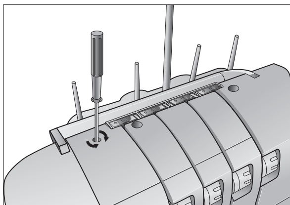
A) Aiguille gauche 5,7 mm
