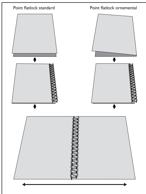
Point flatlock 2 fils
