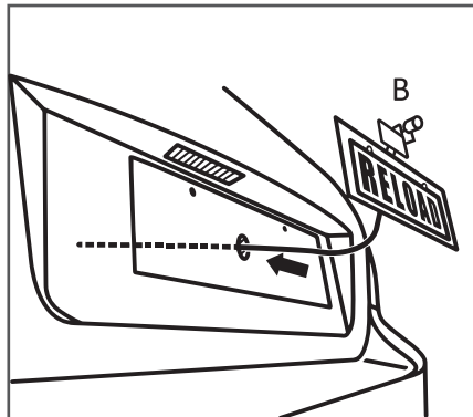
2. Installation de la caméra (B).
