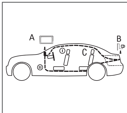
4. Exécution du câble principal (C) du moniteur (A) à l'appareil photo (B).
